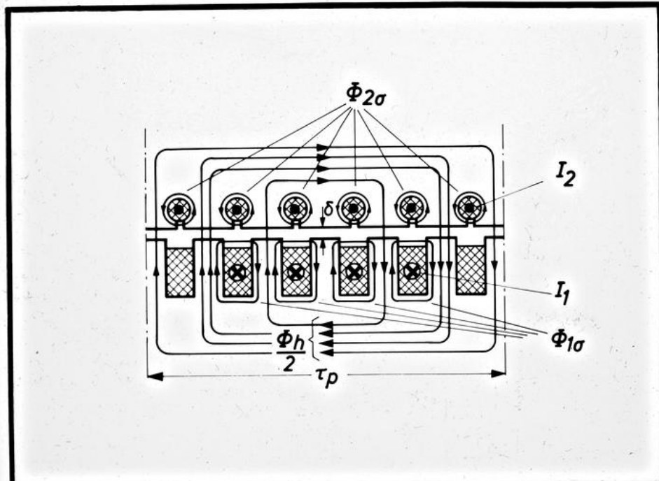
EW THD Hauptfluß und Streuflüsse einer Drehfeldmaschine 0/9.1
