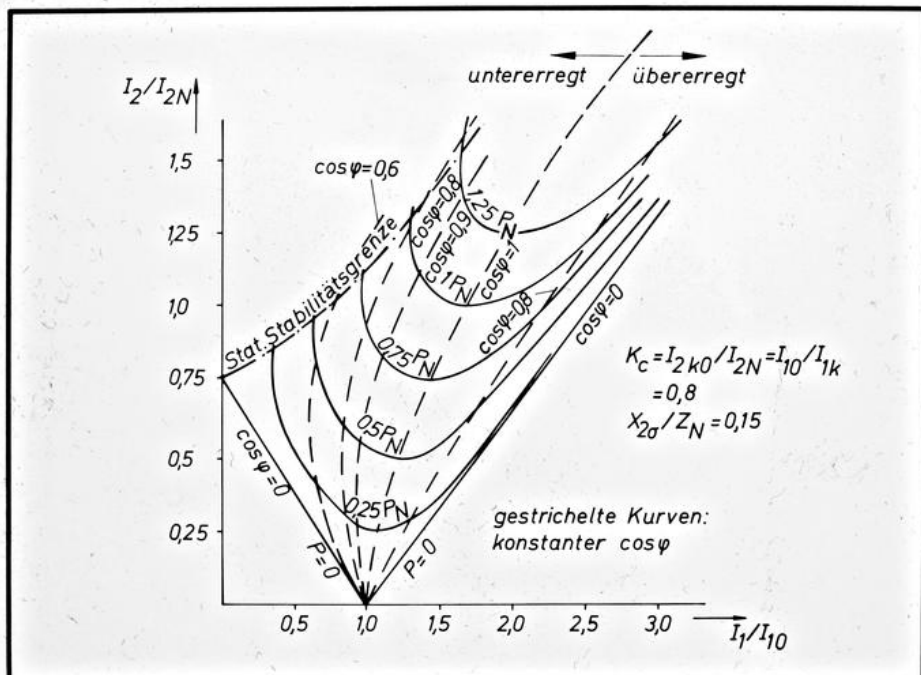
EW V-Kurven und Erregerkurven bei konstanter THD Klemmenspannung und konstanter Wirkleistung 1/9.5
