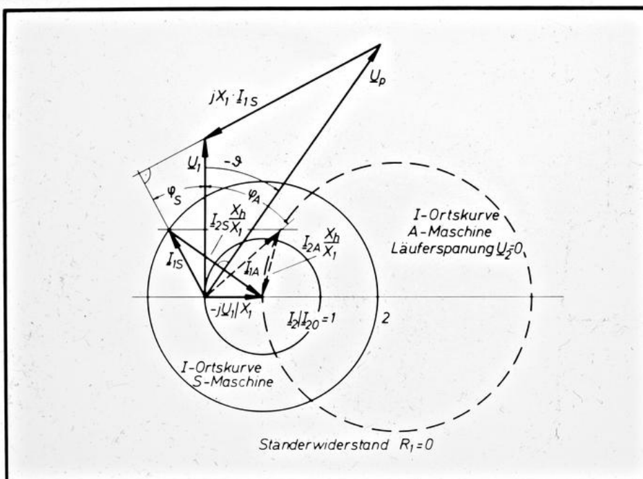
EW Stromortskurven für A-Maschinen mit kurzgeschlos- 2/3.2 THD senem u. mit gleichstromerregtem Schleifringläufer
