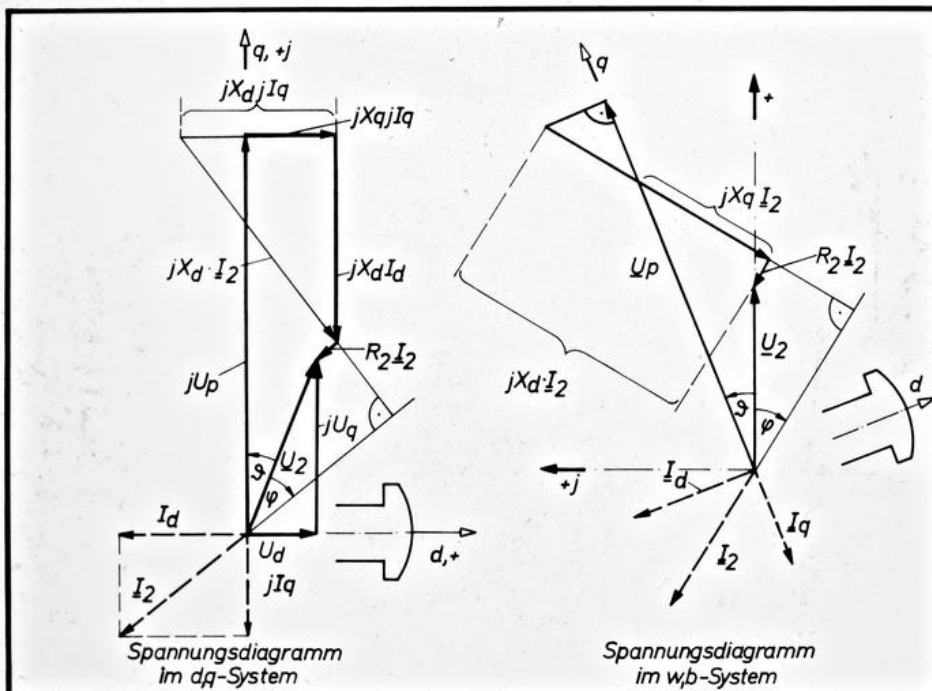
EW Zeigerdiagramm der Synchron-Schenkelpolmaschine, 1/9.1 THD Generatorbetrieb, übererregt
