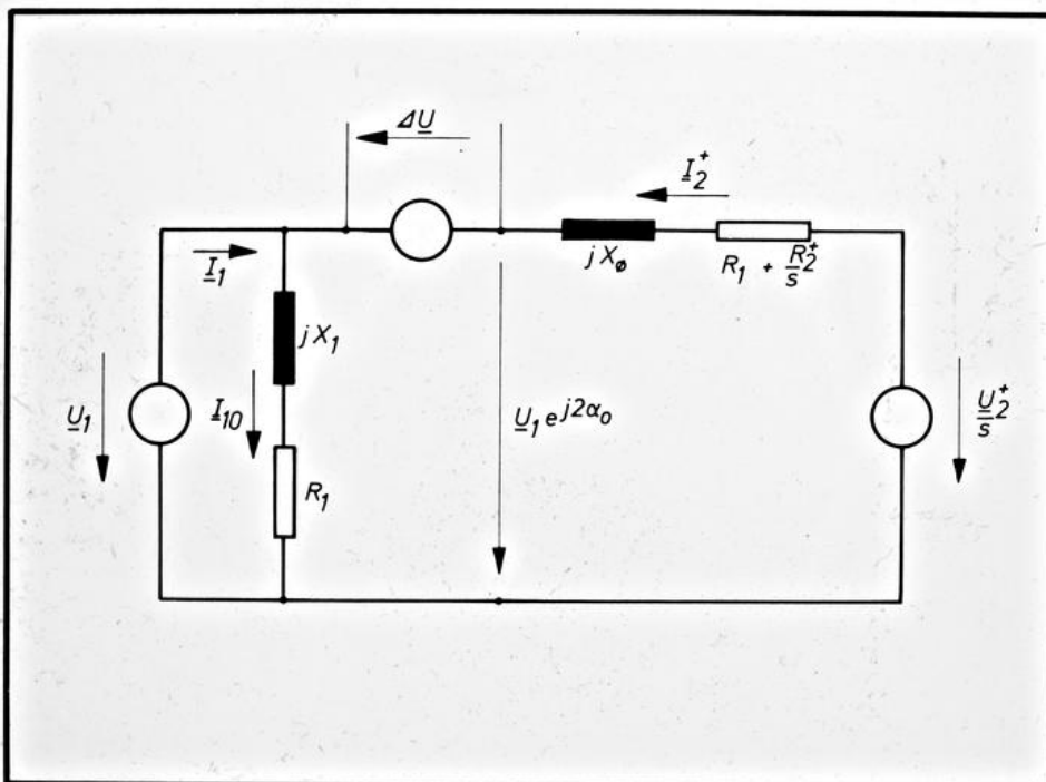
EW THD Ersatzschaltbild der Asynchronmaschine mit komplexem Übersetzungsverhältnis \underline{\dot{u}}_k 1/10.3
