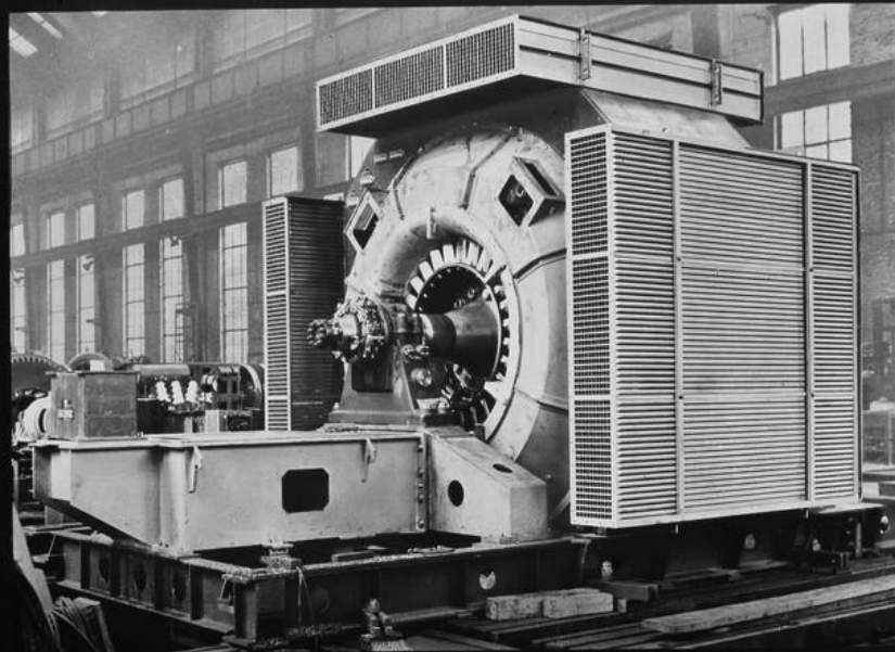
AEG Luftgekühlte Blindleistungsmaschine T \nabla 57 175 000 kVA, 6 600 V, n = 750 U/min 5101
