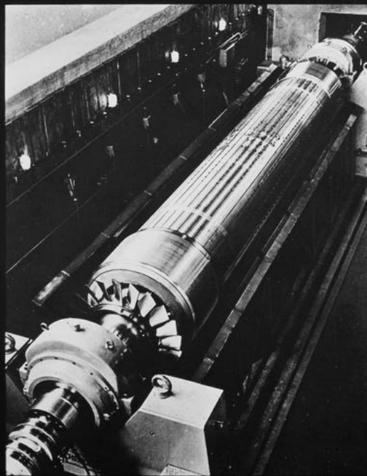
AEG Rotor in der Schleudergrube
