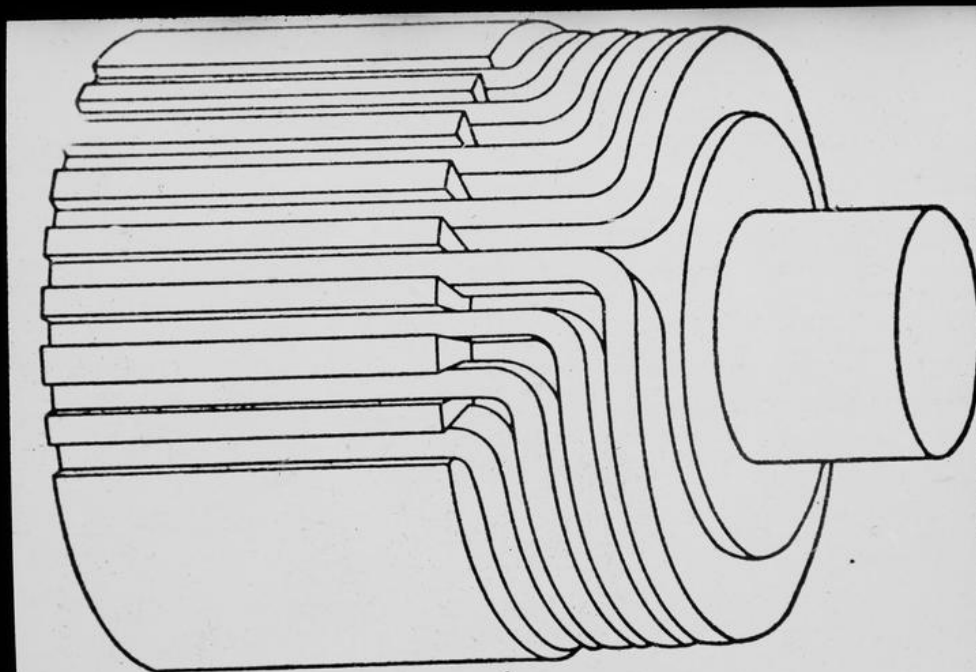
62.3 Zweipolige Läuferwicklung
