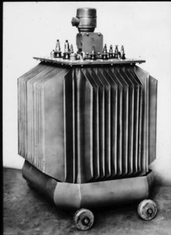
Trockengleichrichtersatz
