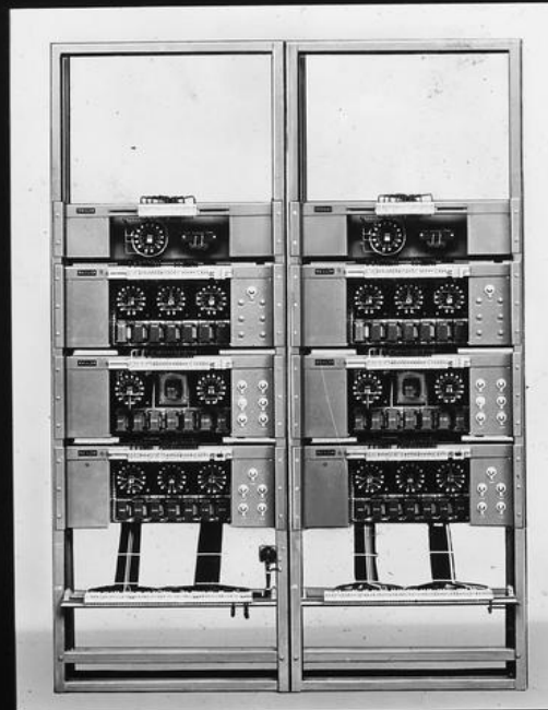
AEG Magnetische Verstärker 400Hz als Regelkreisglieder einer Leonard-Steuerung (Walzwerk-Hauptantriebe)
