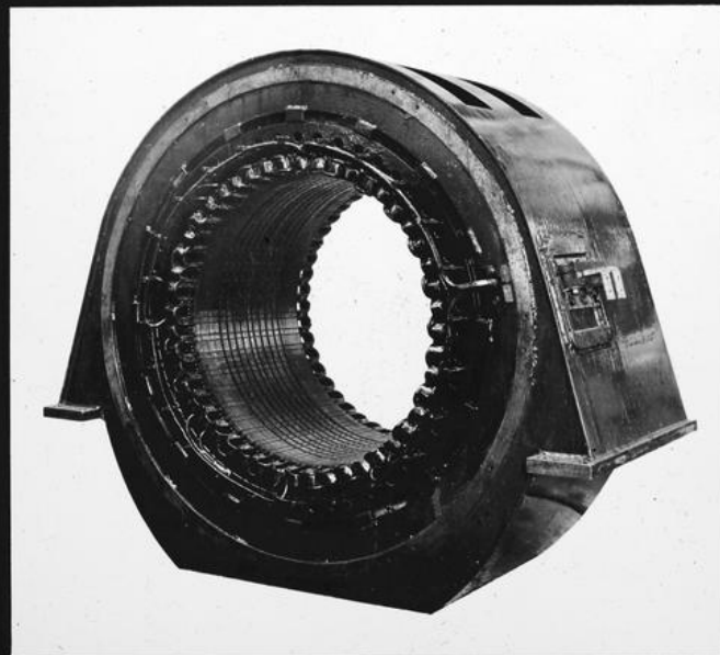
AEG Ständergehäuse mit Wicklung für TV56 Mittelfrequenzgenerator 700 kVA, 600 Hz 2421
