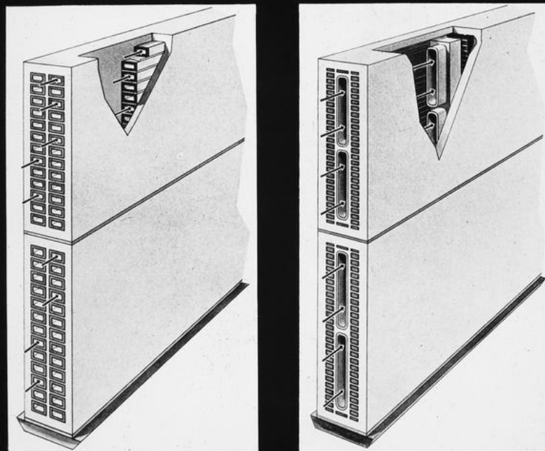
AEG Zwei Ausführungsmöglichkeiten der direkten Kühlung von Ständerwicklungen TV 55 1075
