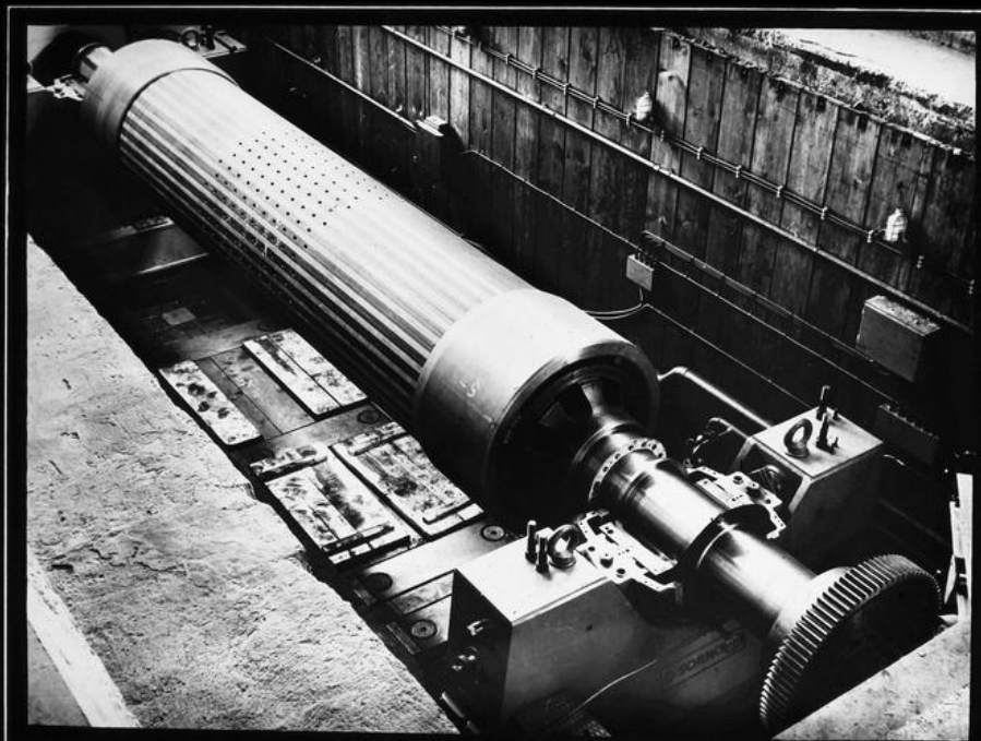
AEG Induktor eines 125 MVA Gen. in TV 1954 der Auswucht- u. Schleudermasch. D32516
