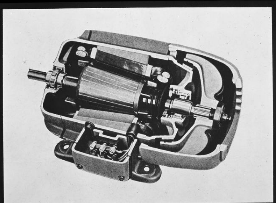
AEG Verschiebeanker-Asynchronmotor TV 57 der DEMAG 4075
