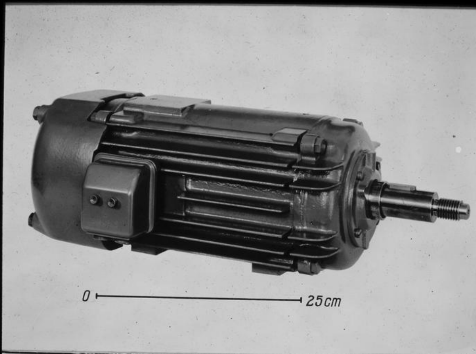
SIEMENS 1950 Kreissägenmotor 3,2 kW, 220/380V, 2860 U/min, Bauform B3 mit Stromdämpfungsläufer G1 500841
