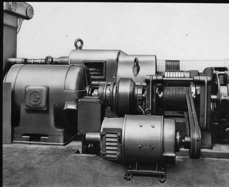
AEG Magnetpulverkupplung EMG zum Antrieb eines Kaltwalzgerüsts TV562830
