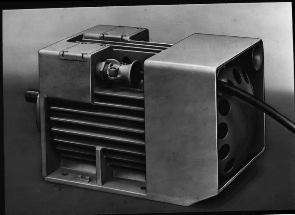
SIEMENS 1956 Druckfester Drehstrom-Asynchronmotor (d UOR 792-4DF) 15 kW, 1500 U/min, bis 500V G1 566709
