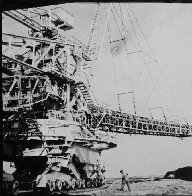
SIEMENS LMG-Absetzer, Bau 162, Roddergrube Berrenrath West G1 1951 30 Motoren, gesamt 1330 kW, 6000/500V~, 440V- 511494
