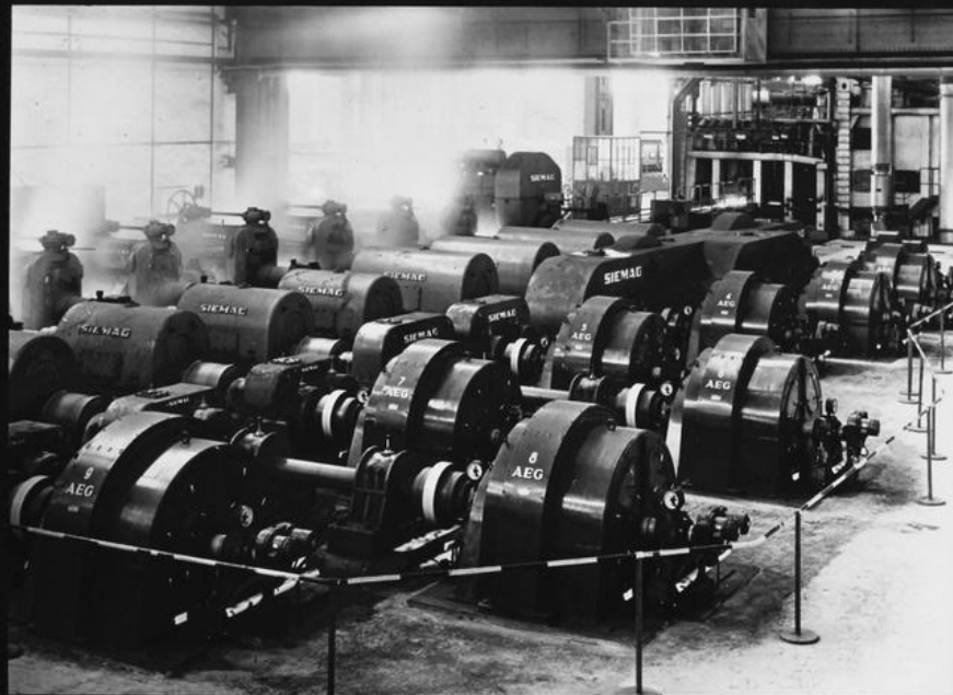
AEG Walzmotoren einer Feisenstraße TV 58 Hüttenwerk Salzgitter AG 6727
