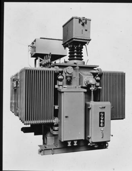
AEG 10/12,5 MVA-Drehstrom-Öltransformator 10 ± 1,35/5,25 kV mit neuen Radiatoren, horizontaler Beblasung u. geräuscharmer Lüfterschachtabdeckung TV 56 3396
