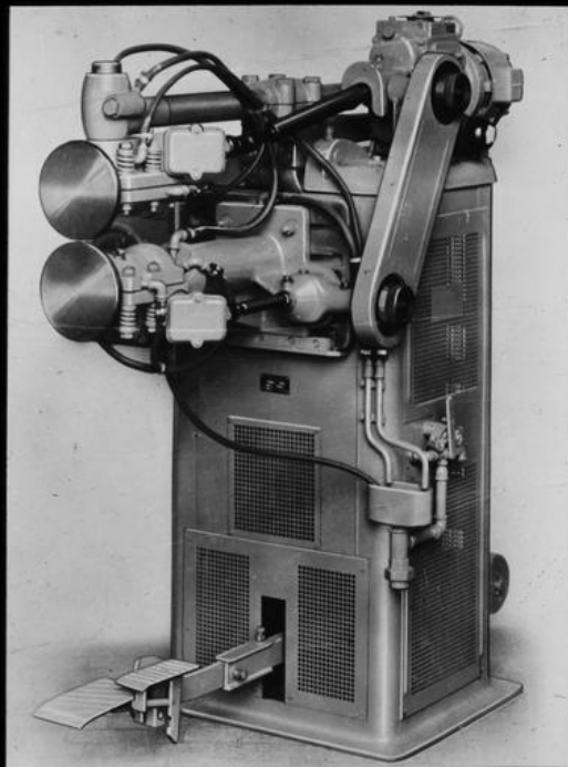
SIEMENS 1949 Hochleistungs-Nahtschweißmaschine (WN 60 Q) mit Doppelrollenantrieb, bis 2×2,5 mm Eisenblech GI 491 128
